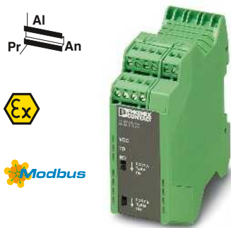
Repetidor para sistemas RS-485 de 2 hilos, separación de 4 vías, ampliable modularmente
