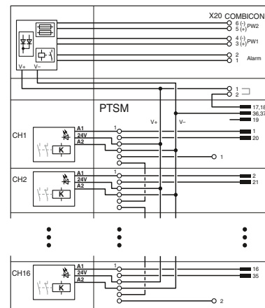
Esquema de conexiones TC-2D37SUB-DO16-F&G-AR-UNI
