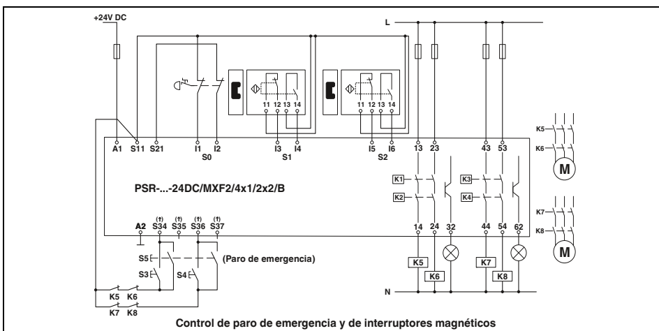
Control de paro de emergencia y de interruptores magnéticos
