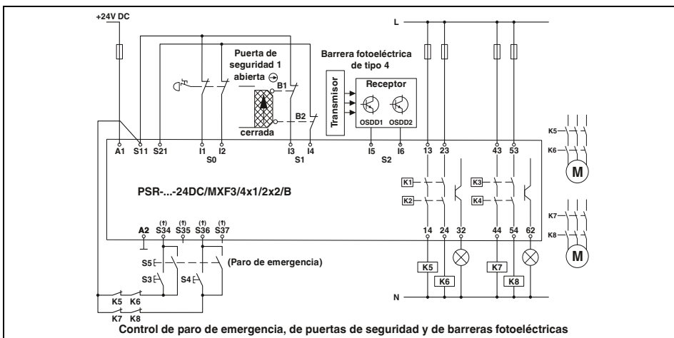
Control de paro de emergencia, de puertas de seguridad y de barreras fotoeléctricas
