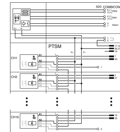
Esquema de conexiones TC-2D37SUB-DO16-ESD-AR-UNI
