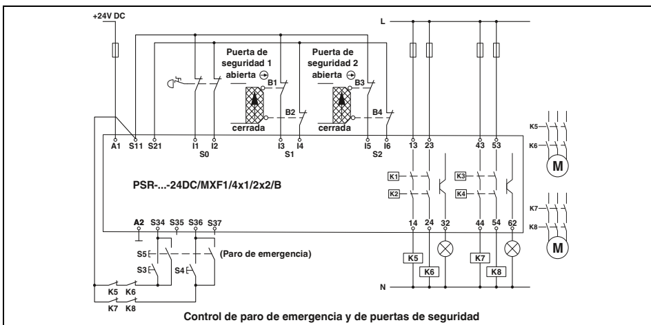
Control de paro de emergencia y de puertas de seguridad
