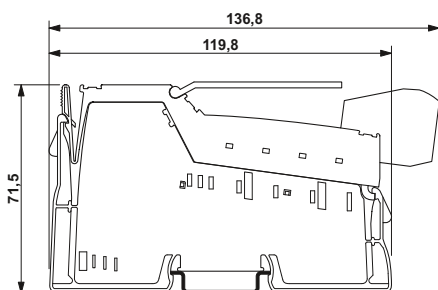
Conector electrónico con conector apantallado
