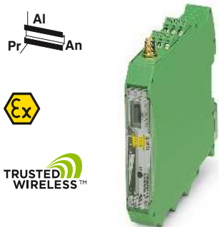
Trasceptor inalámbrico 868 MHz, para el uso sin licencia en Europa
