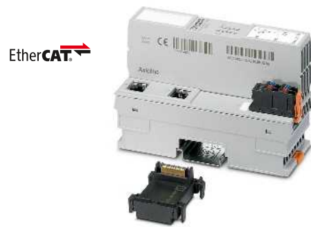
Conexión RJ45
