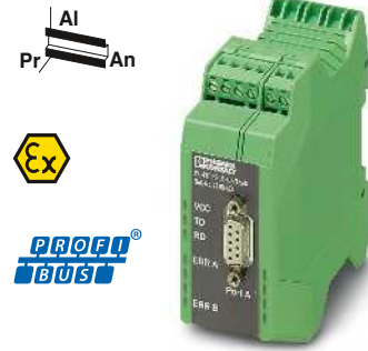
Repetidor para PROFIBUS, separación de 4 vías, ampliable modularmente
