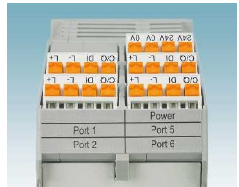
Instalación rápida gracias a la tecnología de conexión push-in
