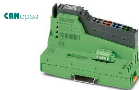
Conexión MINI COMBICON
