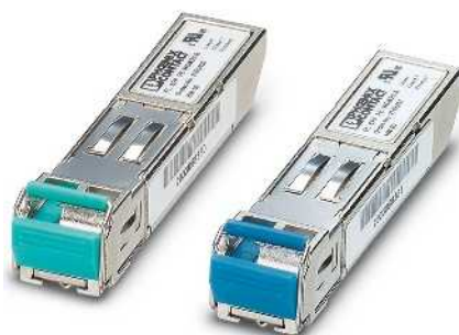
Tecnología WDM, para la transferencia mediante una fibra de vidrio individual
