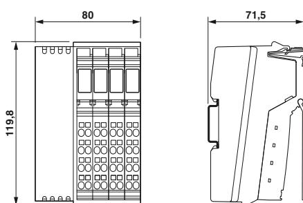
Carcasa BK-IO
