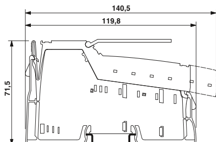
Conector electrónico con conector de señal estándar y doble
