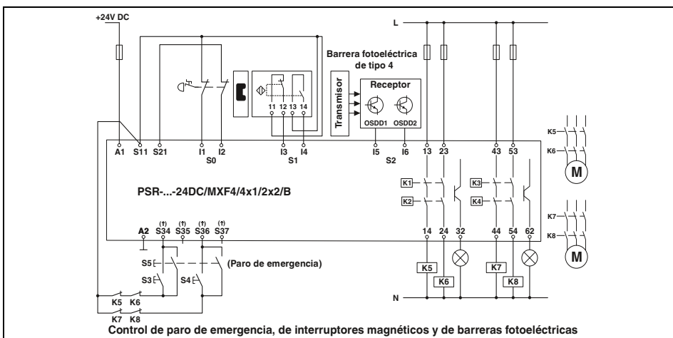
Control de paro de emergencia, de interruptores magnéticos y de barreras fotoeléctricas
