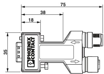
Esquema de dimensiones SUBCON-PLUS...AX...M12, variante axial (180°)
