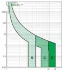
Curvas de disparo Página 9/3
